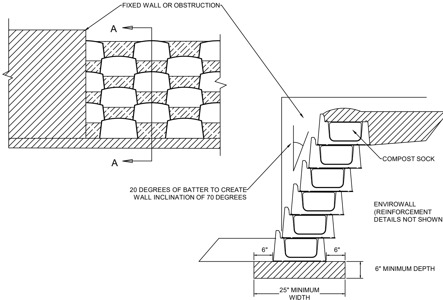
SECTION A-A
